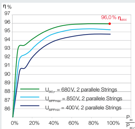
Wirkungsgradkennlinien PIKO 7.0
