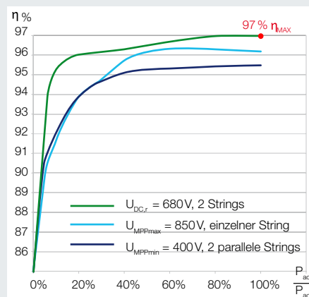
Wirkungsgradkennlinien PIKO 8.3
